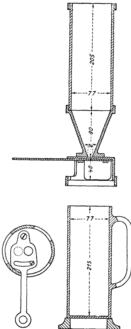
Italian Gravimetro
