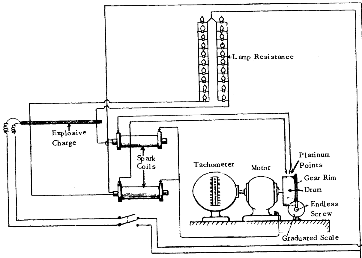
METTEGANG APPARATUS
