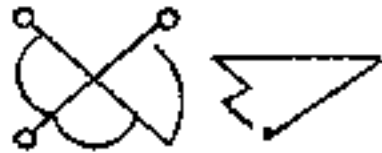
Mars
