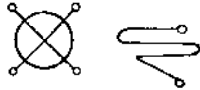
Jupiter
